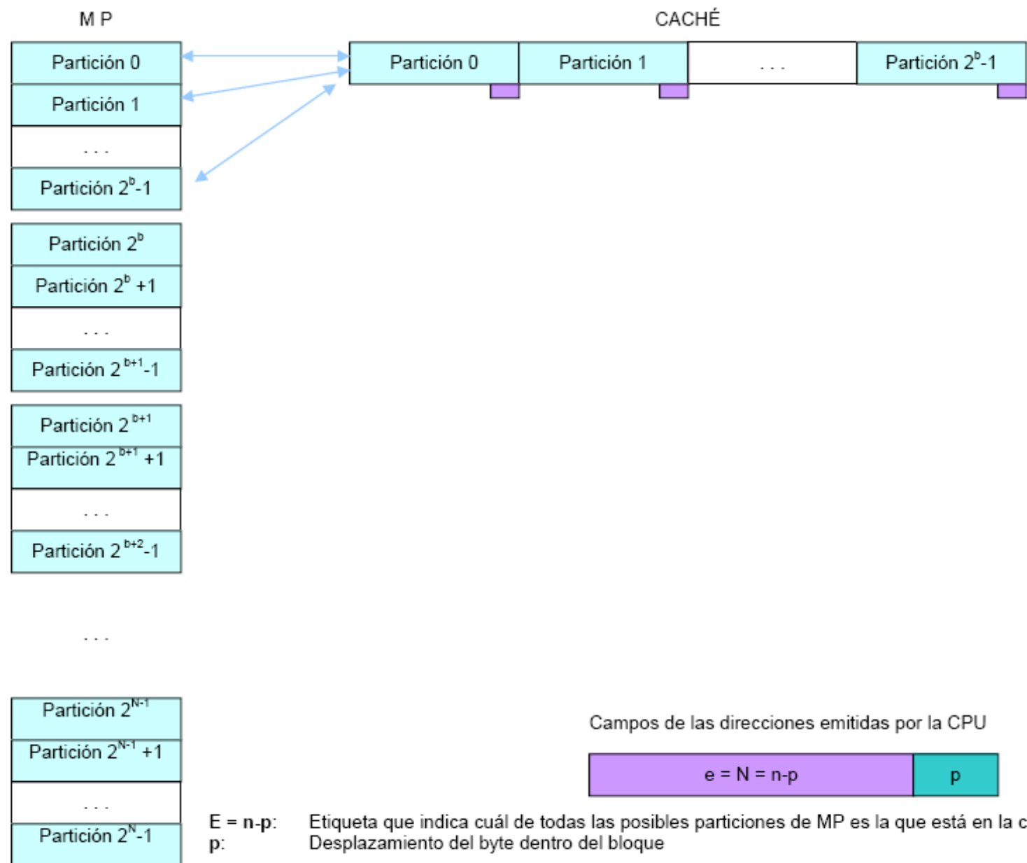
Fig. 15. Asignación de bloques de la M_p en la M_{ca} con correspondencia totalmente asociativa.
