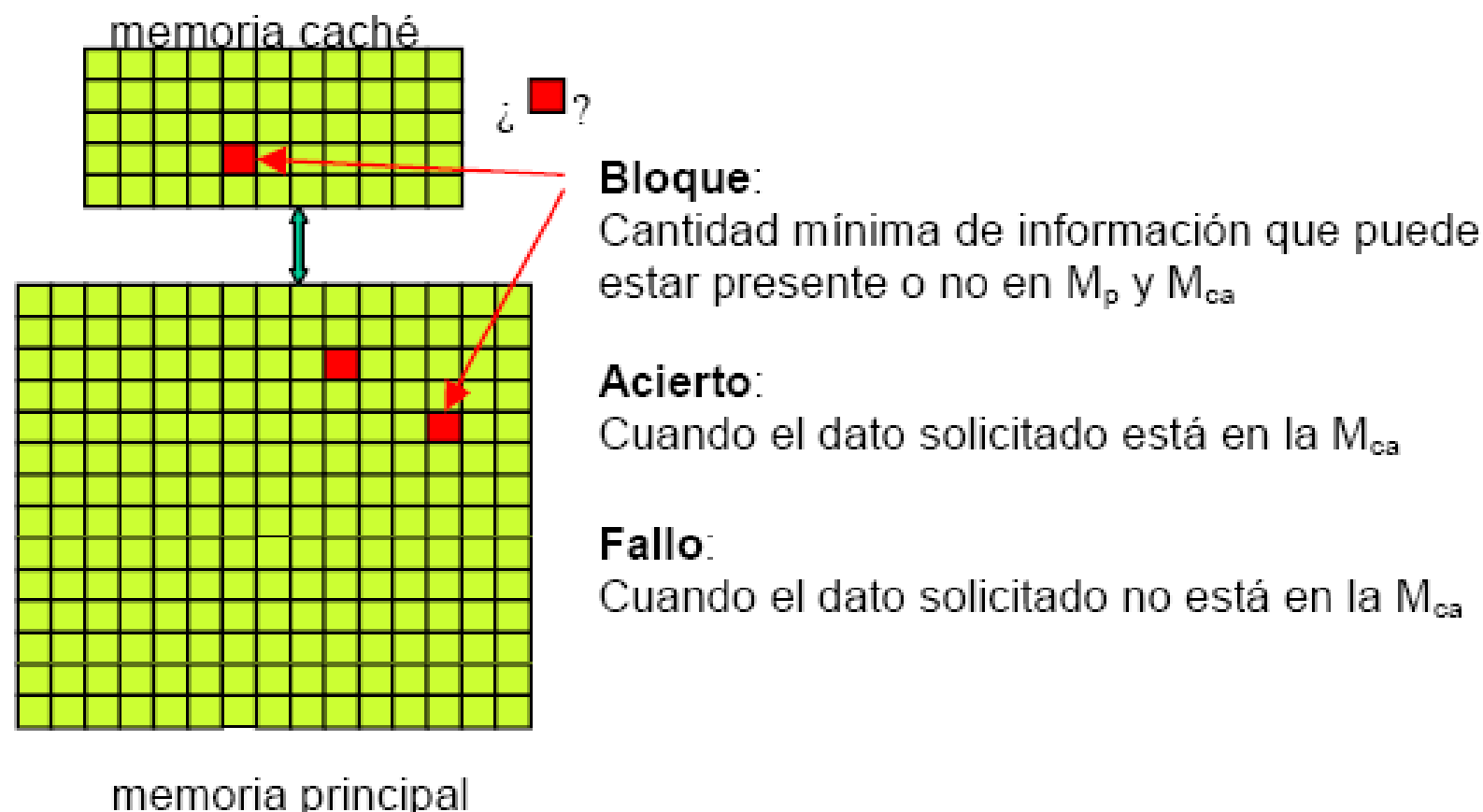
Fig. 03. Conceptos de bloque, acierto y fallo de una memoria caché.
