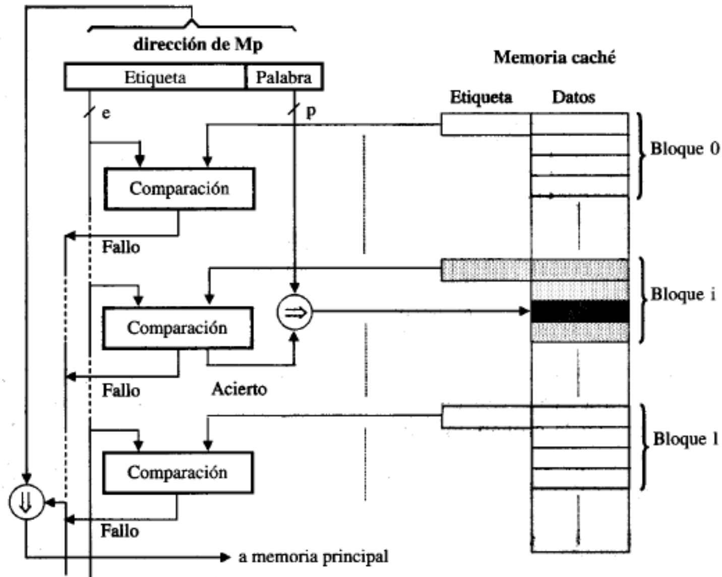
Fig. 16. Organización de una memoria caché con correspondencia totalmente asociativa.
